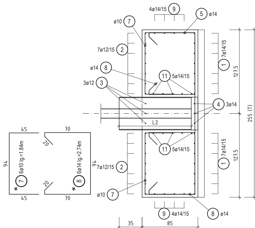
SCHNITT 2-2 M 1:50
