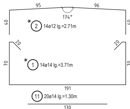
SCHNITT 2-2 M 1:50
