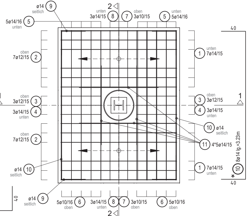
GRUNDRISS M 1:50
