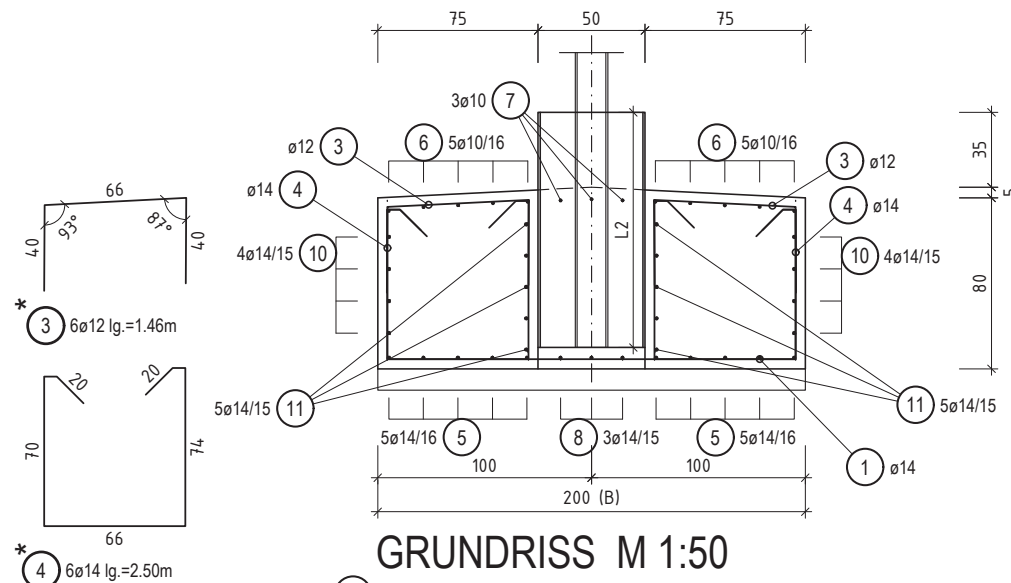
SCHNITT 1-1 M 1:50
